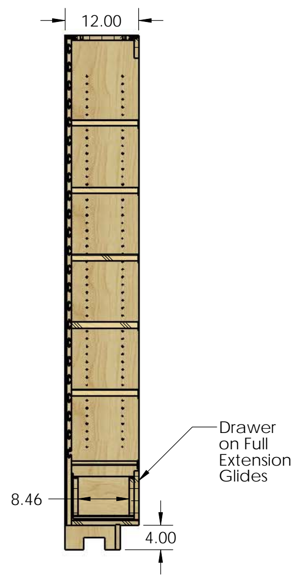
SECTION A-A
