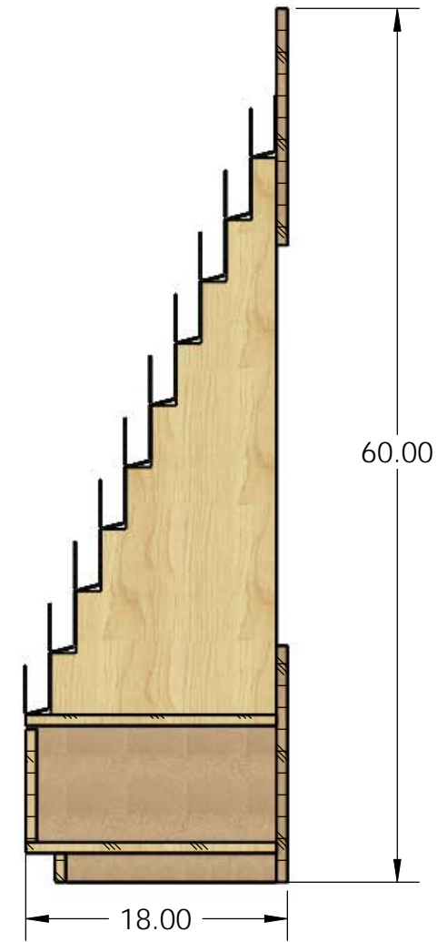
SECTION A-A
